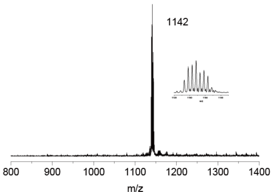
Gd@C 82 Maldi-tof 质谱图
